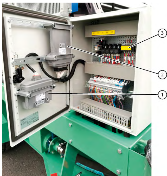
Fig. 16 Armoire électrique
