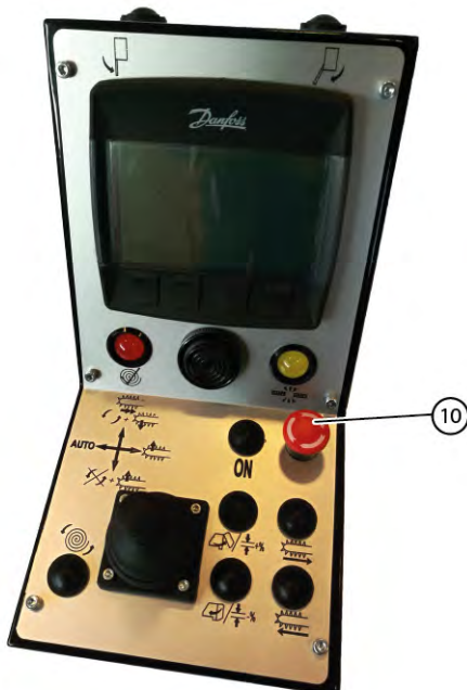
Fig. 54 Arrêter la machine
